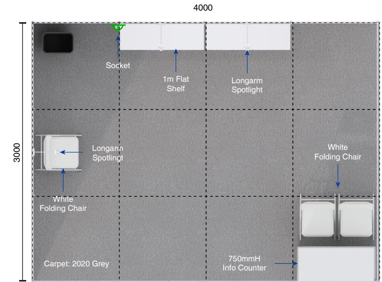
Layout Plan 平面圖
