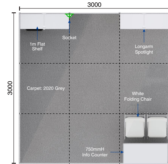
■ Layout Plan 平面圖
